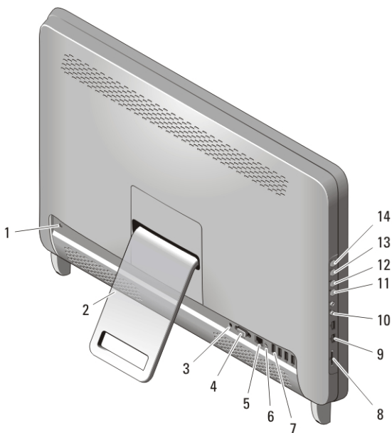
Figura 2. Vista posteriore
